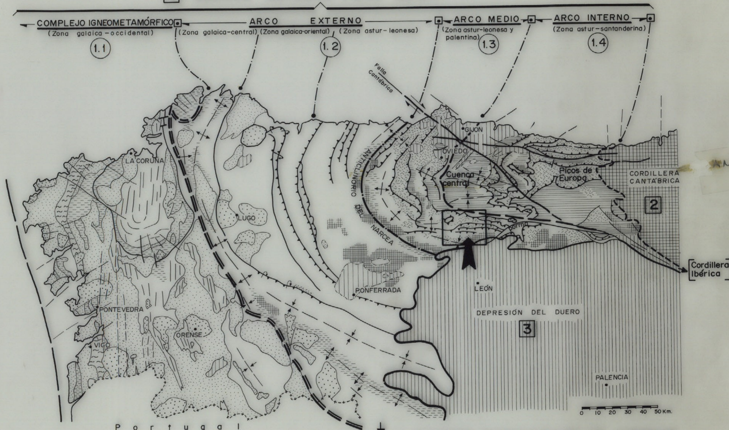
[Meseta] UNIDADES ESTRUCTURALES DEL NOROESTE DE ESPAÑA J. A. Martínez - Álvarez / 1979
