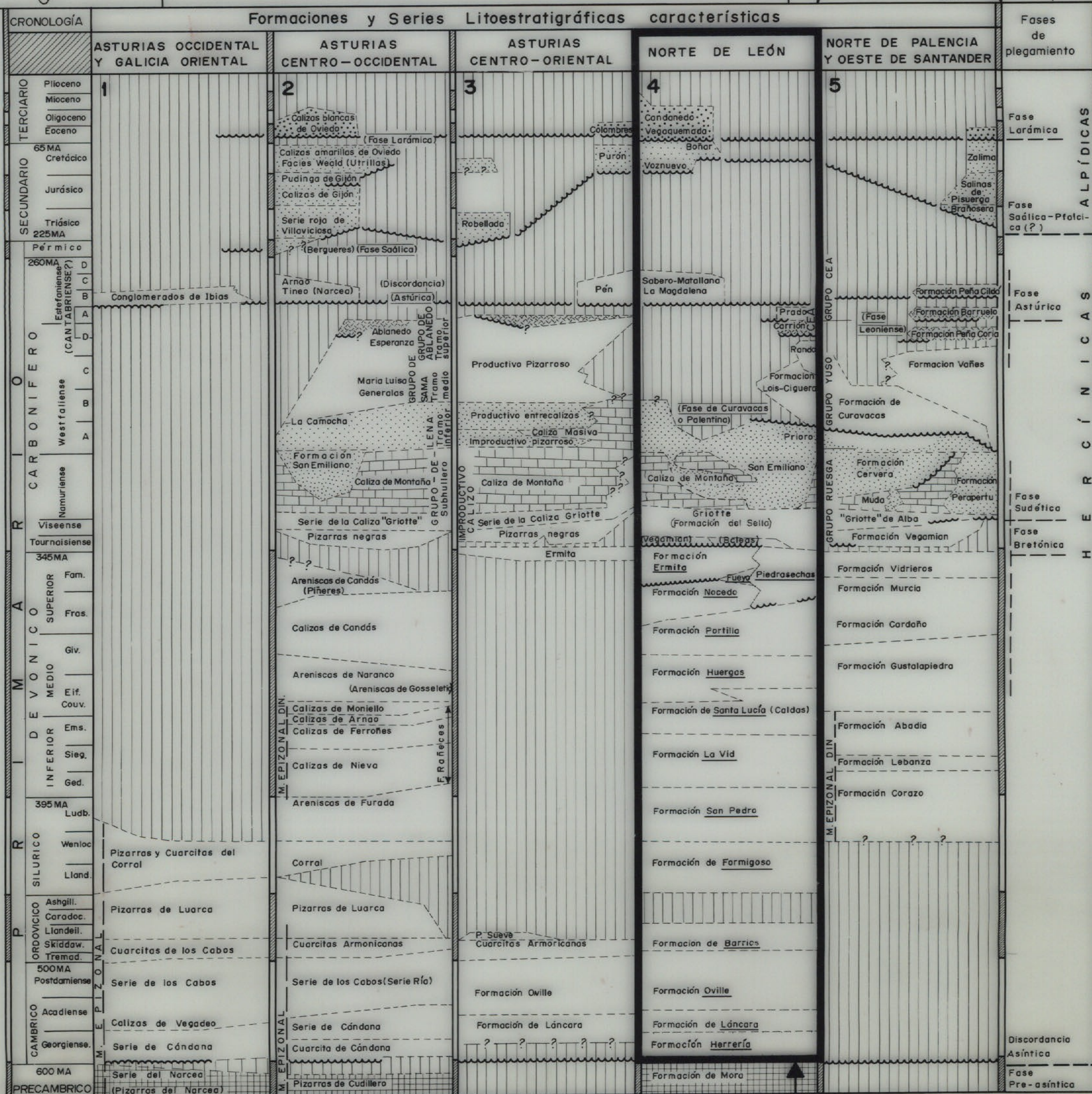
SERIE ESTRATIGRÁFICA CARACTERÍSTICA DEL ÁMBITO DE LA HOJA DE "LA POLA DE GORDON"
